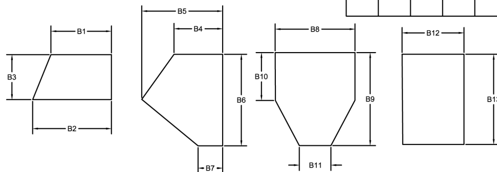
BLADE DIMENSIONS
